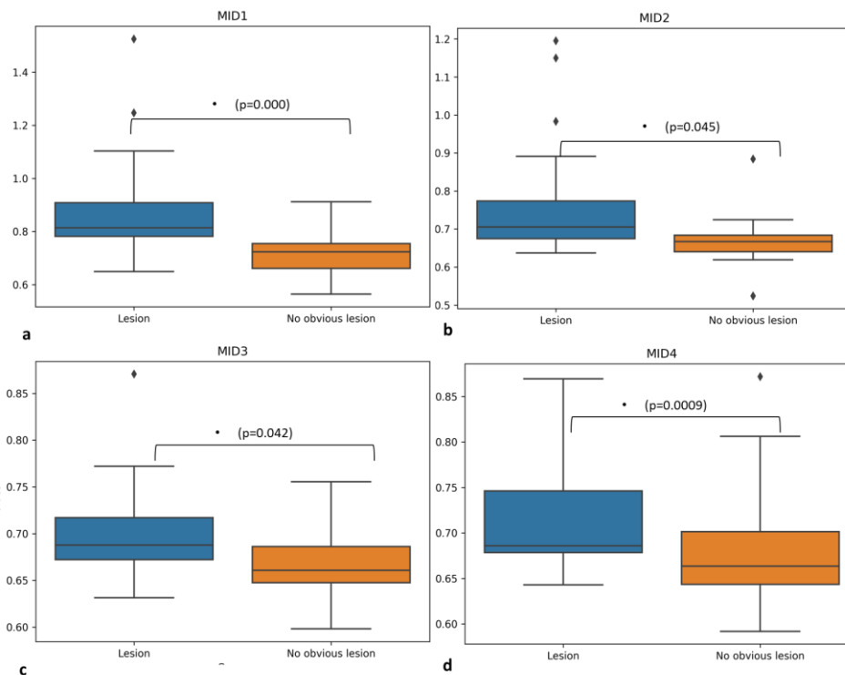
Slika 62. Grafički prikaz srednjih vrijednosti ADC (ordinata, \times 10^{-3} \text{ mm}^2/\text{s} ) i standardnih devijacija kao usporedba između dvogodišnjaka na osnovi prisutnosti perinatalnih lezija u korigiranoj terminskoj dobi. Statistički značajna razlika između navedenih skupina (*, p \leq 0.05 ) prisutna je u središnjem dijelu mozga u vrijednostima svih segmenata.
