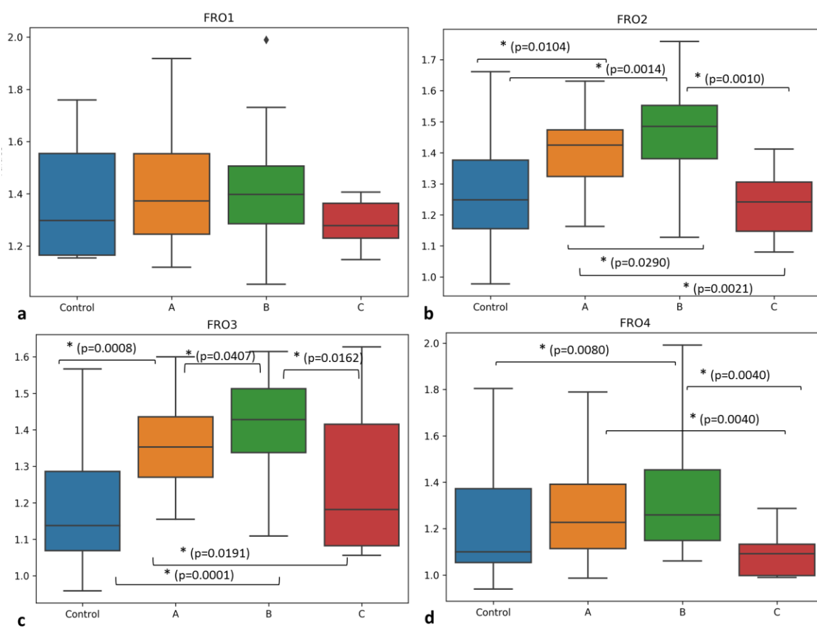
Slika 46. Grafički prikaz srednjih vrijednosti ADC (ordinata, \times 10^{-3} \text{ mm}^2/\text{s} ) i standardnih devijacija u frontalnom dijelu mozga koje se statistički razlikuju međusobno između određenih skupina na temelju različitih segmenata, kako je naznačeno na slici (*, p \leq 0.05 ; A-izrazito nezrela nedonoščad; B- vrlo nezrela nedonoščad; C-kasna do umjerena nedonoščad; Control-novorođenčad rođena u terminu). U segmentu I ne postoje statistički značajne razlike između skupina.
