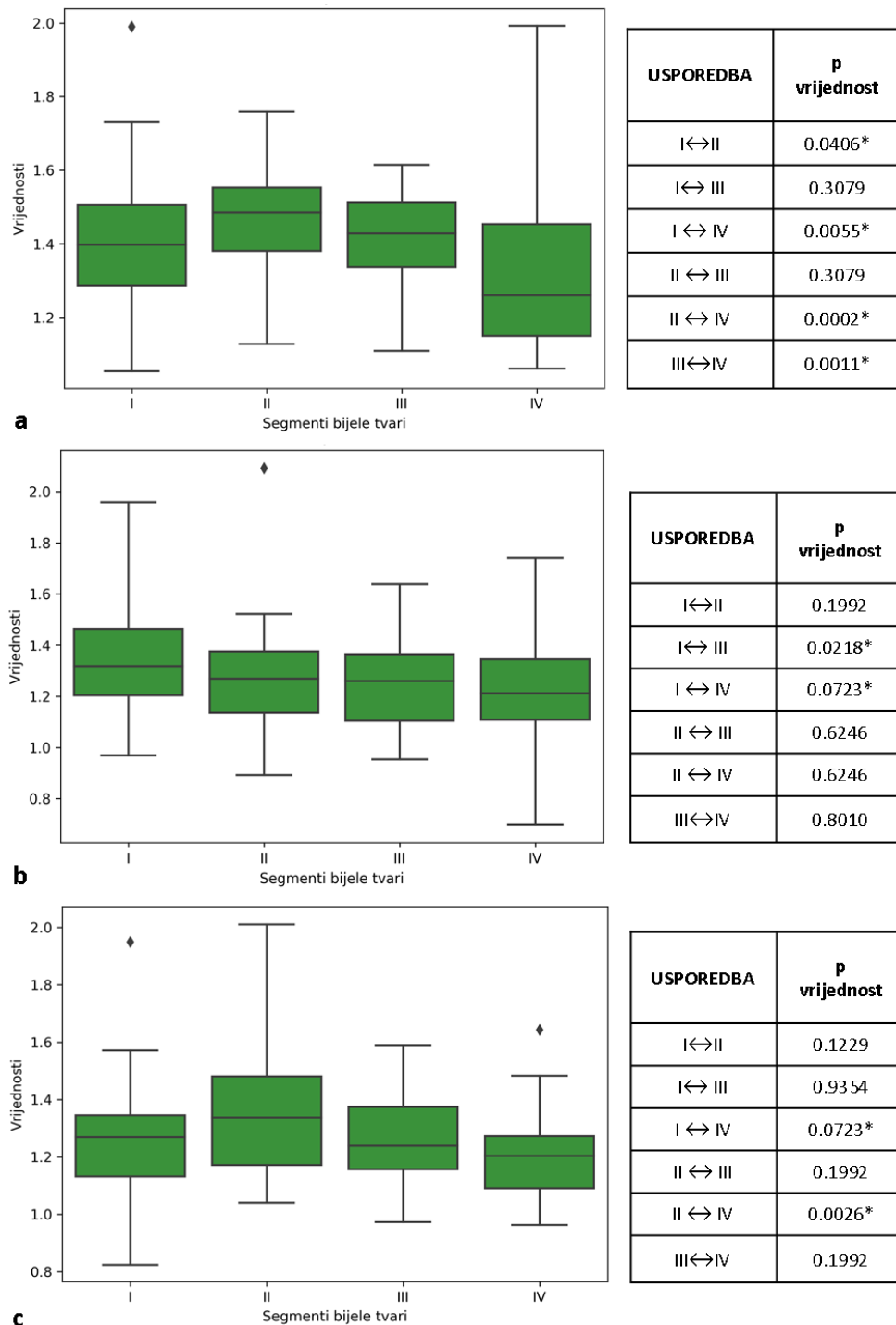
Slika 43. Grafički prikaz srednjih vrijednosti ADC (ordinata, \times 10^{-3} \text{mm}^2/\text{s} ) i standardnih devijacija u skupini umjerene do kasne nedonoščadi po segmentima (apscisa) u različitim dijelovima mozga: frontalno (a), središnje (b), okcipitalno (c). Statistički značajna razlika (*, p \leq 0.05 ) prisutna je frontalno između segmenata I i II, I i IV te II i IV (a). U središnjem dijelu mozga, razlika je statistički značajna između segmenata I i III, te I i IV. U okcipitalnom dijelu mozga, ta razlika je prisutna između segmenata I i IV, te II i IV (c).
