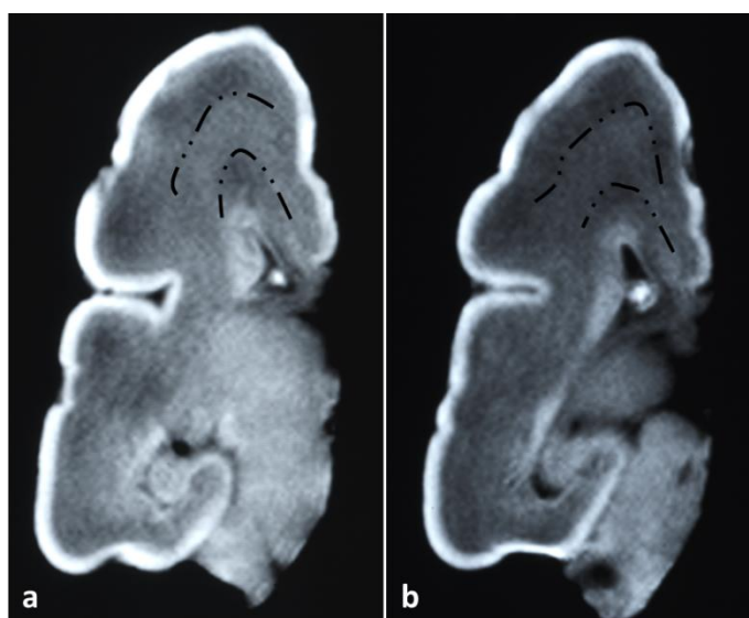
Slika 14. MR in vitro fetalnog mozga gestacijske dobi 24-25 tjedana na kojemu se naziru fetalne zone/budući segmenti na koronarnim presjecima u razini hipokampusu (a) i okcipitalnog reznja (b). Saggittal strata nemaju jasno podijeljenje slojeve.
