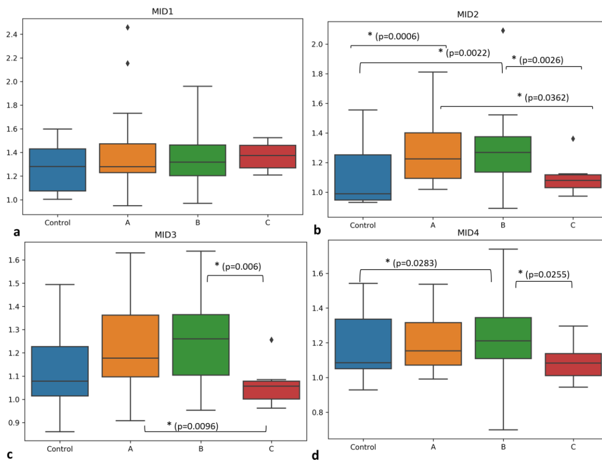
Slika 47. Grafički prikaz srednjih vrijednosti ADC (ordinata, \times 10^{-3} \text{mm}^2/\text{s} ) i standardnih devijacija u frontalnom dijelu mozga koje se statistički razlikuju međusobno između određenih skupina na temelju različitih segmenata, kako je naznačeno na slici (*, p \leq 0.05 ; A-izrazito nezrela nedonoščad; B- vrlo nezrela nedonoščad; C-kasna do umjerena nedonoščad; Control-novorodenčad rođena u terminu). U segmentu I ne postoje statistički značajne razlike između skupina.
