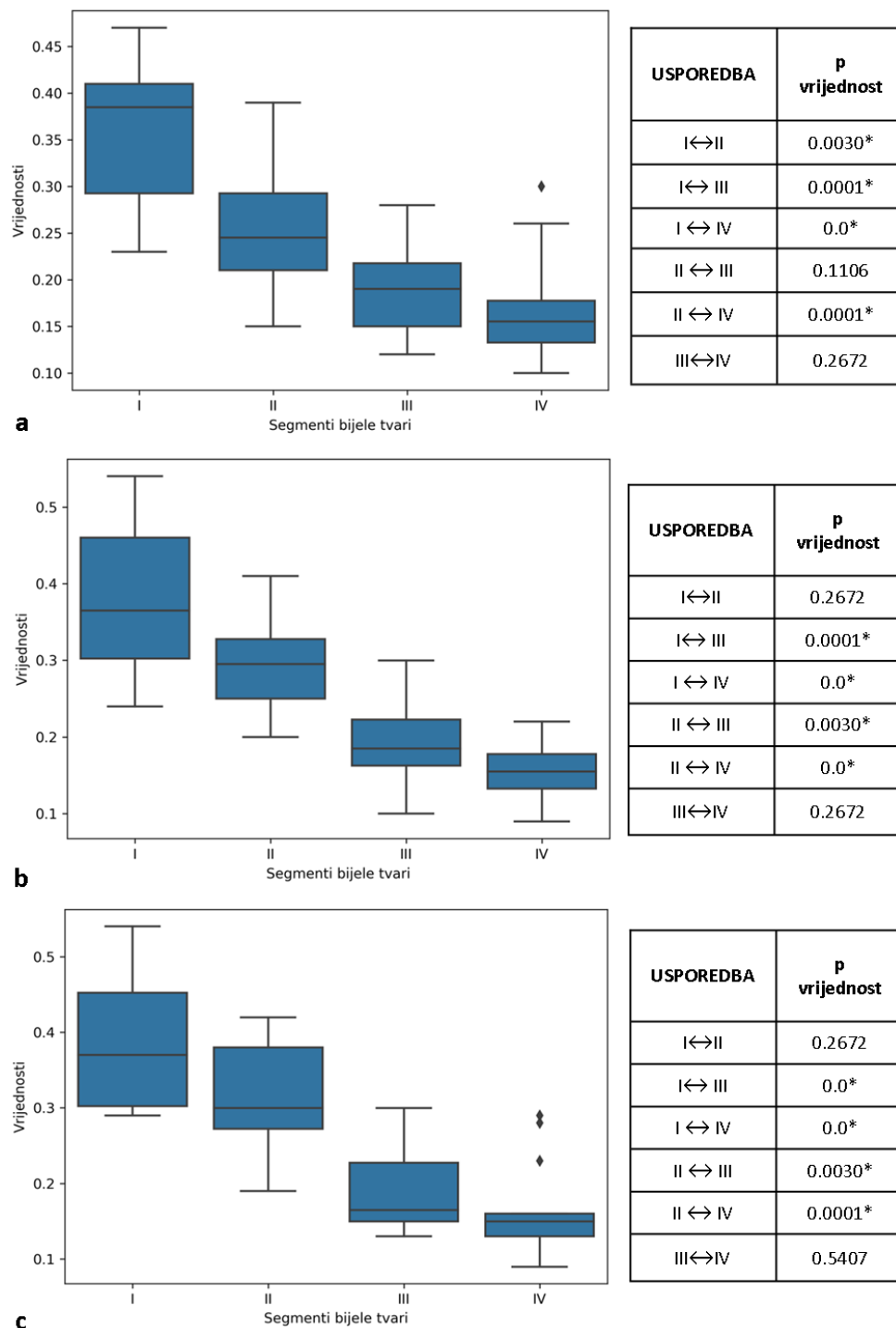
Slika 35. Grafički prikaz srednjih vrijednosti FA (ordinata) i standardnih devijacija u skupini terminske novorođenčadi po segmentima (apscisa) u različitim dijelovima mozga: frontalno (a), središnje (b), okcipitalno (c). Statistički značajna razlika (*, p \leq 0.05 ) prisutna je međusobno između svih segmenata u različitim istraživanim područjima (a, b, c), osim frontalno između segmenata II i III; III i IV (a); centralno između segmenata I i II, te III i IV (b); i okcipitalno između segmenata I i II, III i IV (c).
