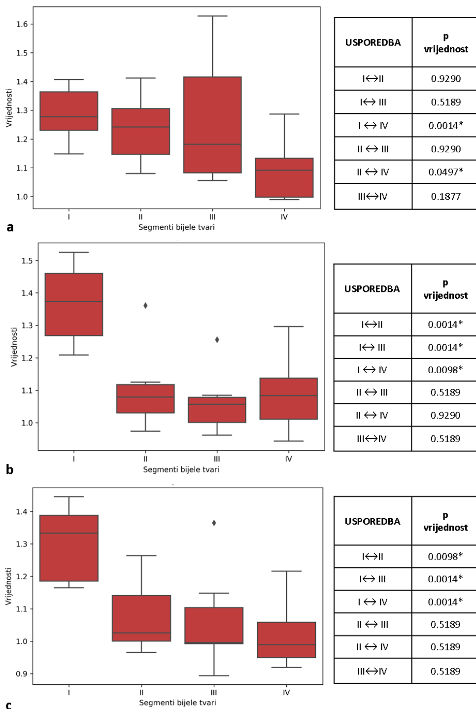
Slika 44. Grafički prikaz srednjih vrijednosti ADC (ordinata, \times 10^{-3} \text{mm}^2/\text{s} ) i standardnih devijacija u skupini vrlo nezrele nedonoščadi po segmentima (apscisa) u različitim dijelovima mozga: frontalno (a), centralno (b), okcipitalno (c). Statistički značajna razlika ( p \leq 0.05 ) prisutna je frontalno između segmenata I i IV te II i IV (a). U središnjem dijelu, razlika je značajna između segmenata I i II, I i III te I i IV (b); dok u okcipitalnom dijelu mozga, razlika je najznačajnija između segmenata I i III te I i IV (c).
