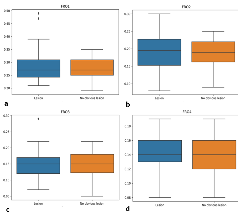
Slika 39. Grafički prikaz srednjih vrijednosti FA (ordinata) i standardnih devijacija u području segmenata I-IV u frontalnom režnju. Nema statistički značajne razlike između nedonošćadi koji su imali perinatalne lezije na MR nalazu (engl. lesion) i onih koji nisu imali očitih lezija na MR nalazu (engl. no obvious lesion).
