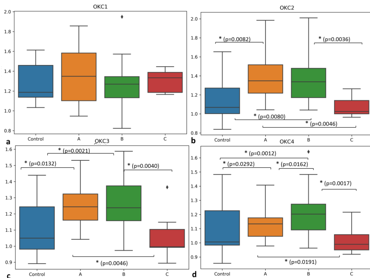
Slika 48. Grafički prikaz srednjih vrijednosti ADC (ordinata, \times 10^{-3} \text{ mm}^2/\text{s} ) i standardnih devijacija u frontalnom dijelu mozga koje se statistički razlikuju međusobno između određenih skupina na temelju različitih segmenata, kako je naznačeno na slici (*, p \leq 0.05 ; A-izrazito nezrela nedonoščad; B- vrlo nezrela nedonoščad; C-kasna do umjerena nedonoščad; Control-novorodjenčad rođena u terminu). U segmentu I ne postoje statistički značajne razlike između skupina.
