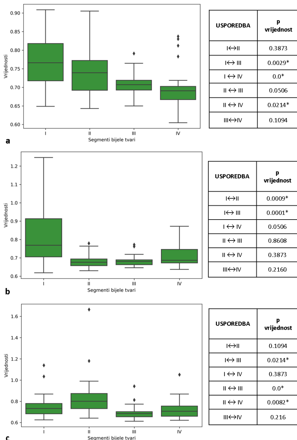
Slika 56. Grafički prikaz srednjih vrijednosti ADC (ordinata, \times 10^{-3} \text{ mm}^2/\text{s} ) i standardnih devijacija u skupini dvogodišnjaka rođenih kao vrlo nezrela nedonoščad (apscisa) u različitim dijelovima mozga: frontalno (a), središnje (b), okcipitalno (c). Statistički značajna razlika (*, p \leq 0.05 ) prisutna je između segmenata I i III, I i IV, II i IV frontalno (a), segmenata I i II, te I i III u središnjem dijelu mozga dok je u okcipitalnom dijelu (c) ta razlika prisutna između segmenata I i III, II i III te II i IV.
