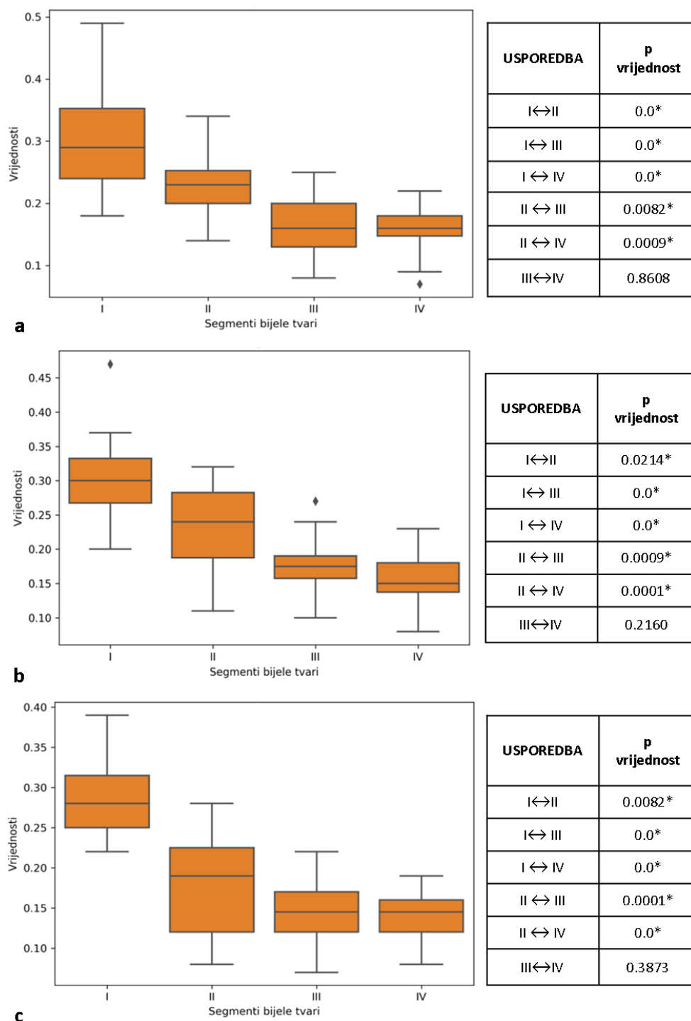
Slika 32. Grafički prikaz srednjih vrijednosti FA (ordinata) i standardnih devijacija u skupini izrazito nezrele nedonoščadi po segmentima (apscisa) u različitim dijelovima mozga: frontalno (a), središnje (b), okcipitalno (c). Statistički značajna razlika (*, p \leq 0.05 ) prisutna je međusobno između svih segmenata u svim istraživanim područjima mozga, osim između segmenata III i IV.
